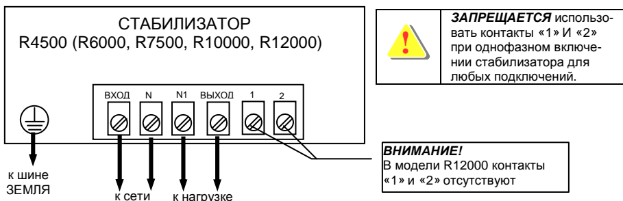
Рисунок 6.1 Схема подключения стабилизатора
